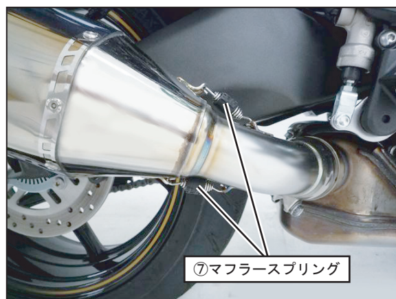
8. 車両後方から見てサイレンサーの傾きやマフラーと車両との距離を調整し、クランプバンド、純正ボルト、ボタンボルトM6の順に仮締めしていたボルト、ナットを規定トルクで締め付けて下さい。 (F I G. 10. 11参照)
