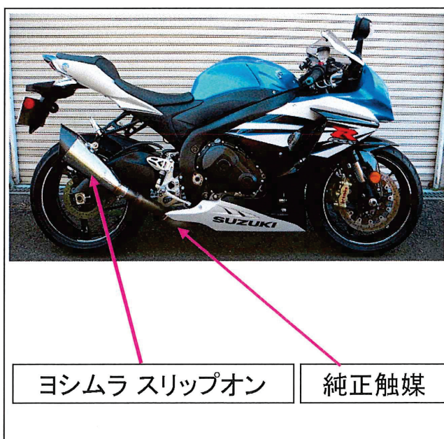
製品と純正触媒の取付写真
